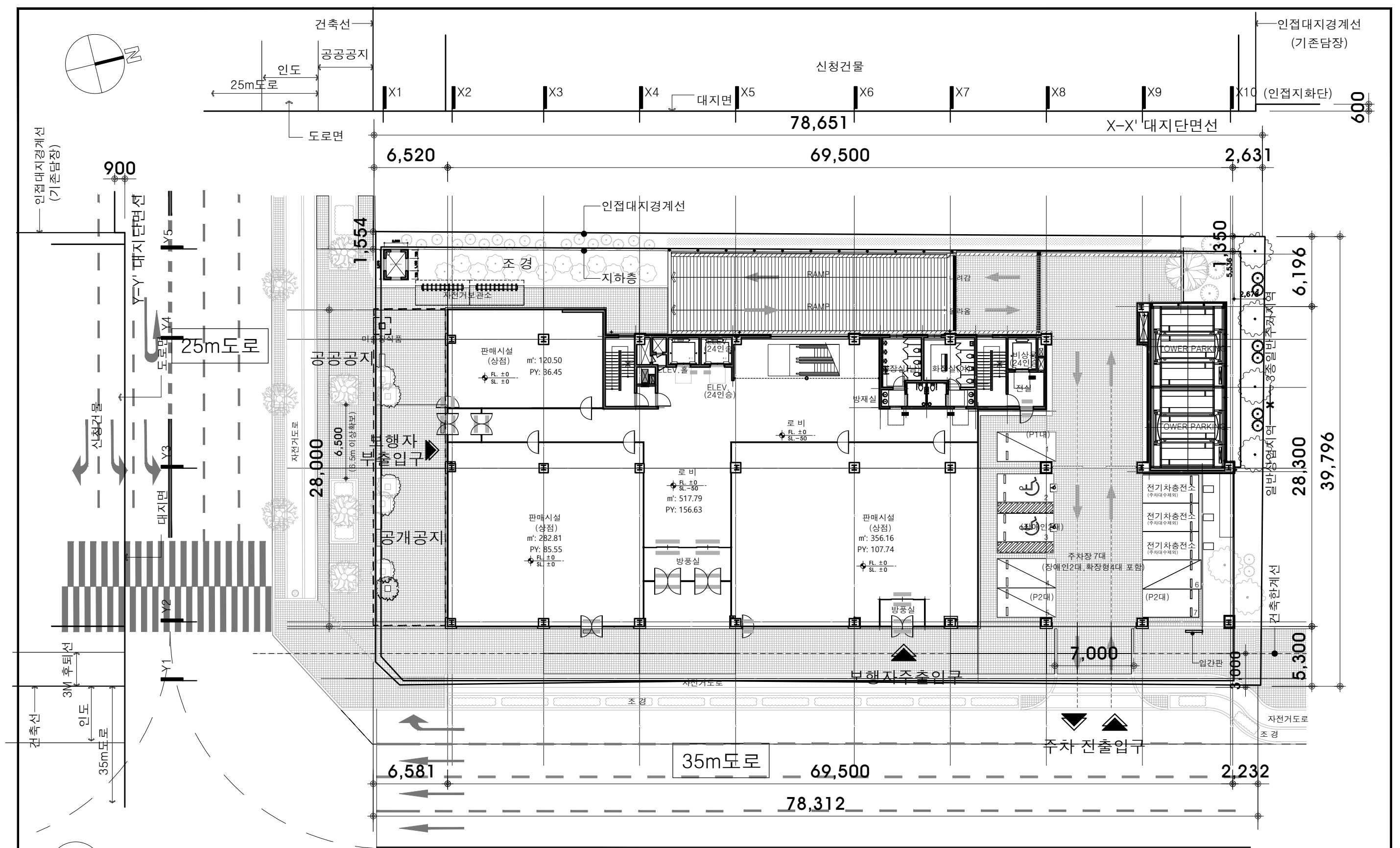
배치도 SCALE - A3 : 1/300
